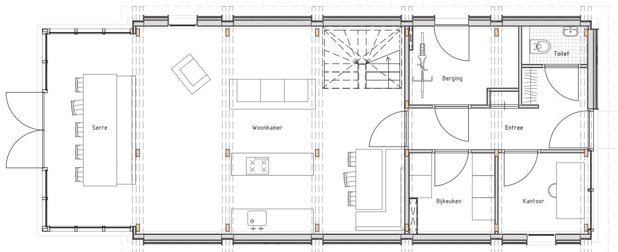
Plattegrond eerste verdieping
