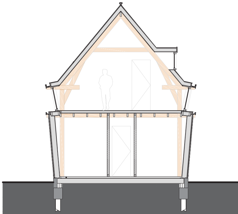
Doorsnede Fortwachterswoning
